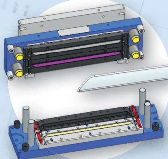
OUTIL D'EMBOSSAGE & DECOUPAGE SEUIL AUTOMOBILE
